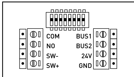
Detailsicht Anschlusspanel
