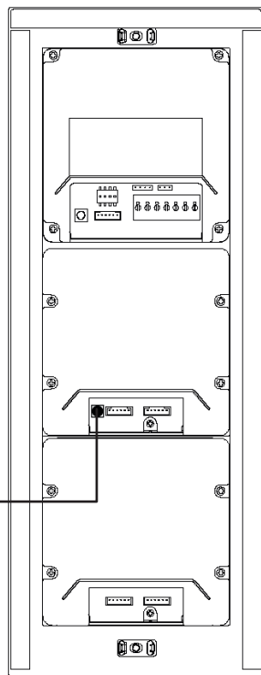
EVO-6FAM-RFID Rückseite
